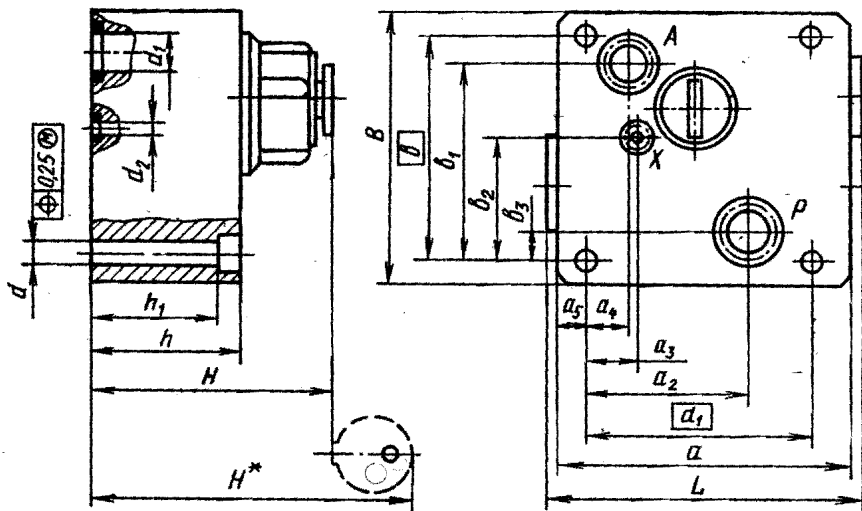
Рис. 168. Габаритные и присоединительные размеры регуляторов расхода с обратным клапаном типа МПГ55-3.М:
