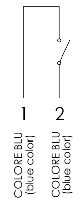
SCHEMA ELETTRICO (electric scheme)
