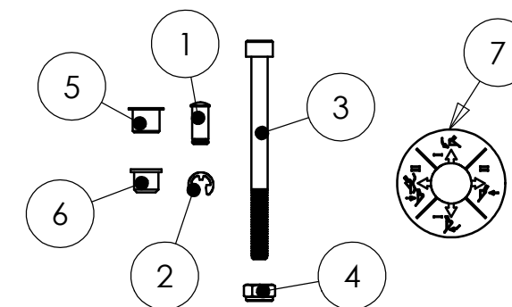
KIT FISSAGGIO CAVI (631128) (cable fixing kit 631128)
